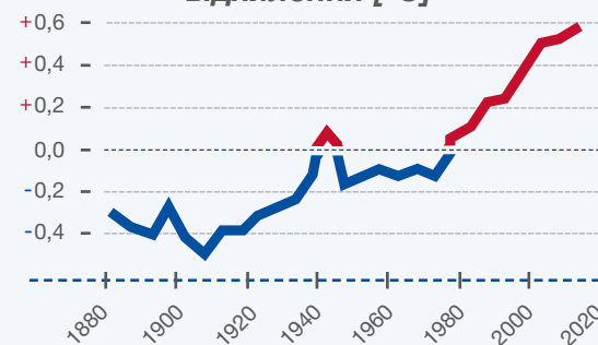
Глобальне підвищення середнього показника температури, відхилення [°C]
