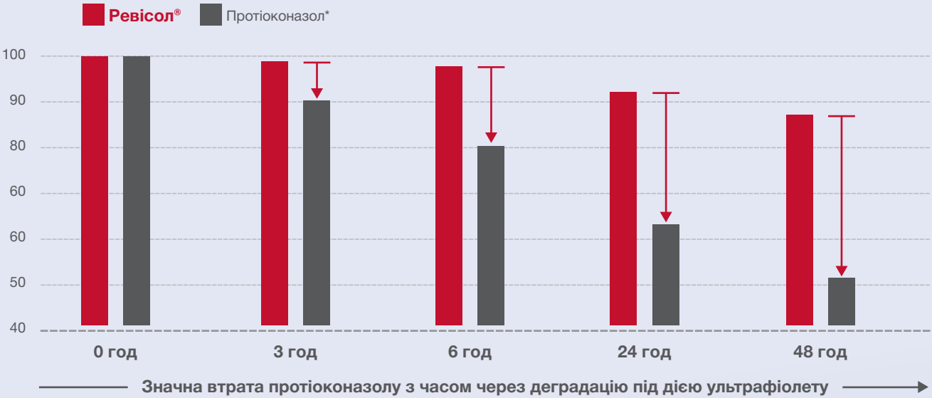
Кількісне визначення Ревісол® порівняно з протіоконазолом* впродовж певного періоду, дослід з використанням сонячного тестера [% від початкової кількості]
