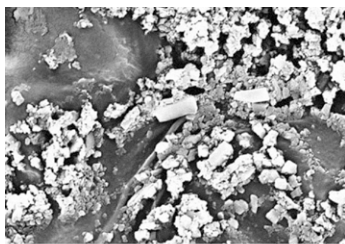
BAS 669 010007 2012/08/03 11:35 H D9.8 x4.0k 20 um 1.2L/ha 600L Apfel 7d + Wasser
